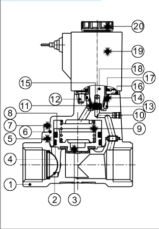
2WA150 (Grommet)
